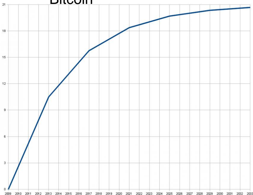
График эмиссии Bitcoin
